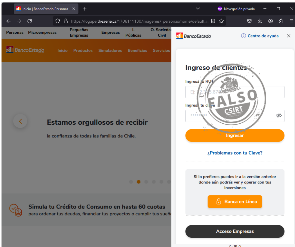
Imagen 2: Sitio fraudulento
